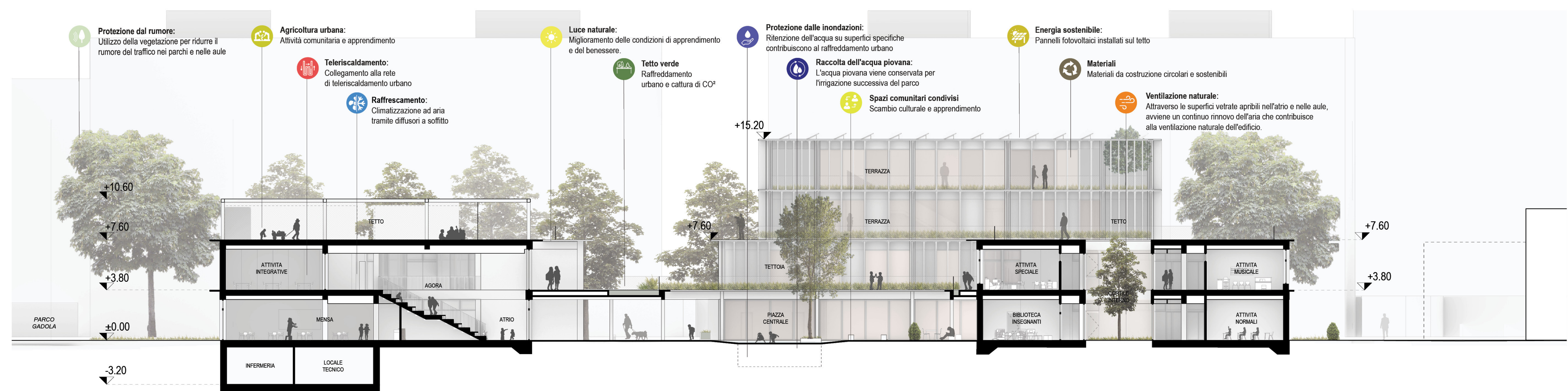
SEZIONE BB' SOSTENIBILITÀ | 1:200 | IL COMMUNITY CAMPUS
