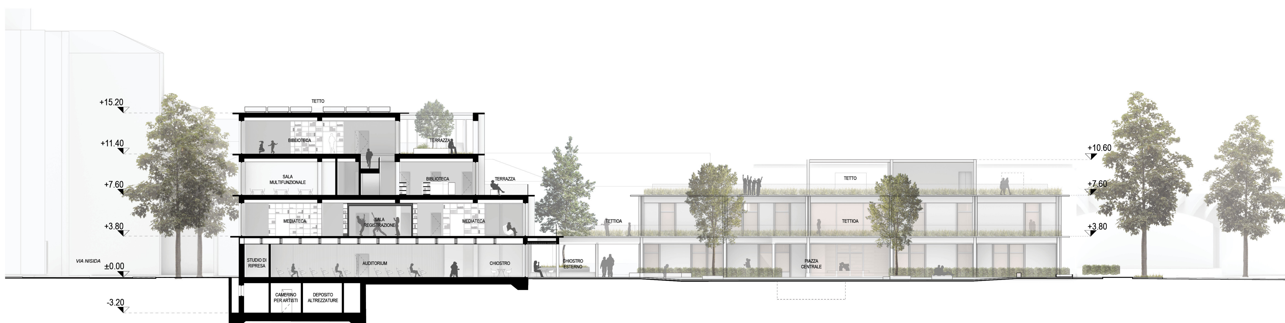
SEZIONE AA' | 1:200 | IL COMMUNITY CAMPUS
